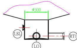
液出口示意圖
